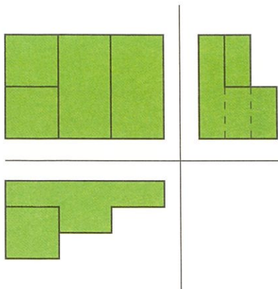
Proiezioni ortogonali
